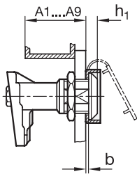
Türverriegelung GN 119
