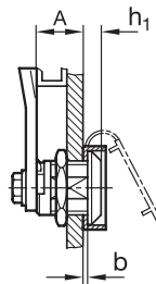
Verriegelungen GN 115
